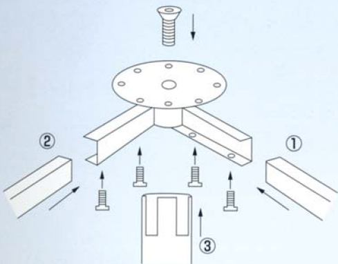
<組立図>
